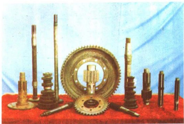
▲图为县农机修造一厂开发生产的农用机械齿轮，轴类零配件。
