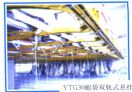
YTG30邮袋双轨式悬挂输送机
