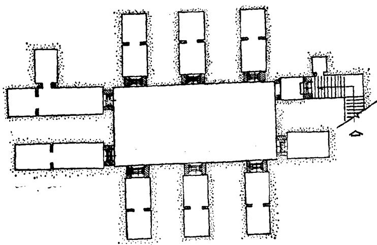
图 5 天井院式的窑洞
