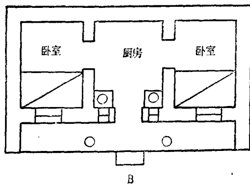
图 3 华北农村住宅
