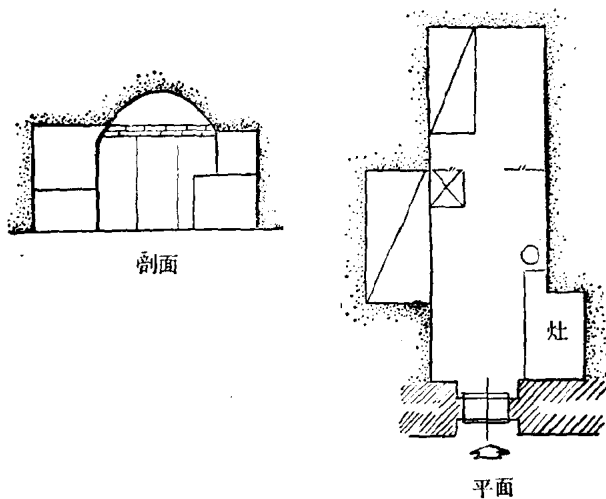
图 4 黄土高原地区的窑洞建筑
