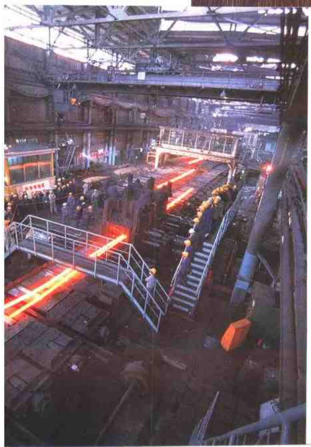
首钢初轧厂初 轧切分轧制
