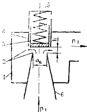
图2—1 安全阀示意图
