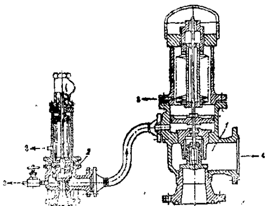
图2—2 先导式安全阀示例
