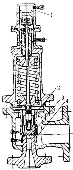
图2-3 带补充载荷的安全阀
