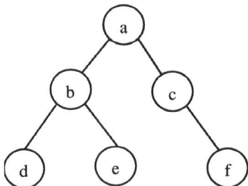
图 1.1 一棵二叉树
