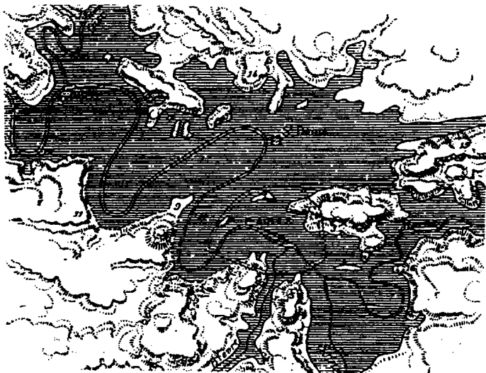
古代巴黎地区地理状况图（约200万年前）
