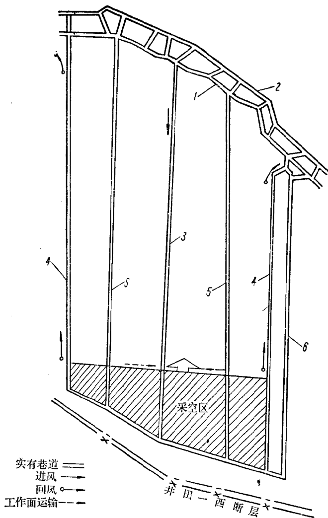
图 1-3 田屯矿471工作面倾斜条带巷道布置
