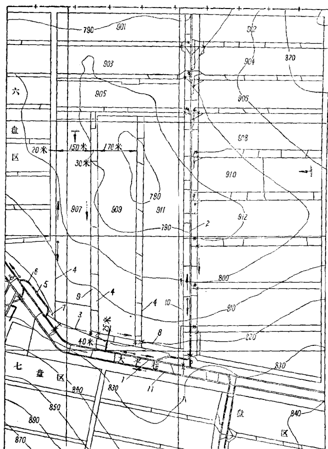
图 1-2 阳泉一矿北头嘴九盘区改造布置
