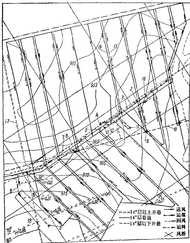
图 1-1 永定庄矿西一盘区14#层巷道布置
