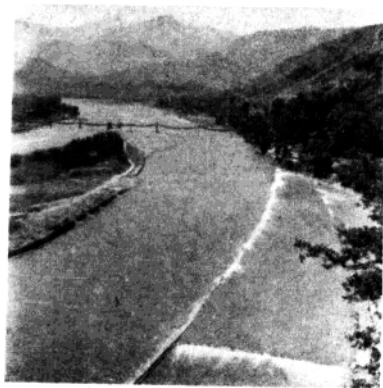
照片3 都江堰及索桥, 桥下为内外江分水鱼嘴 (张吉年摄, 人民画报社稿)
