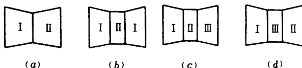
图 1-2 导流分期与围堰分段示意图
