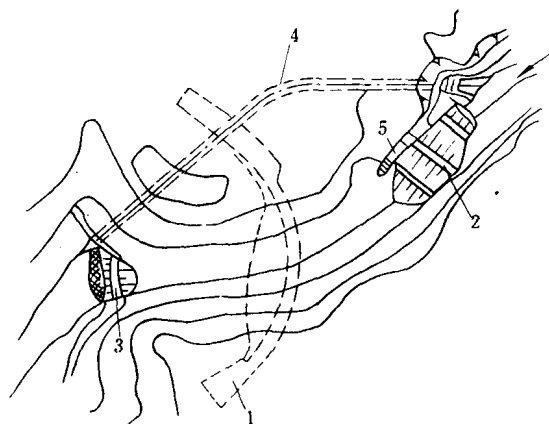
图 1-6 青海省龙羊峡水电站隧洞导流
