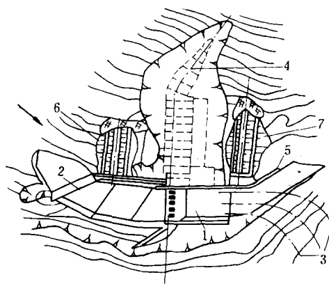
图 1-5 天生桥二级水电站工程
