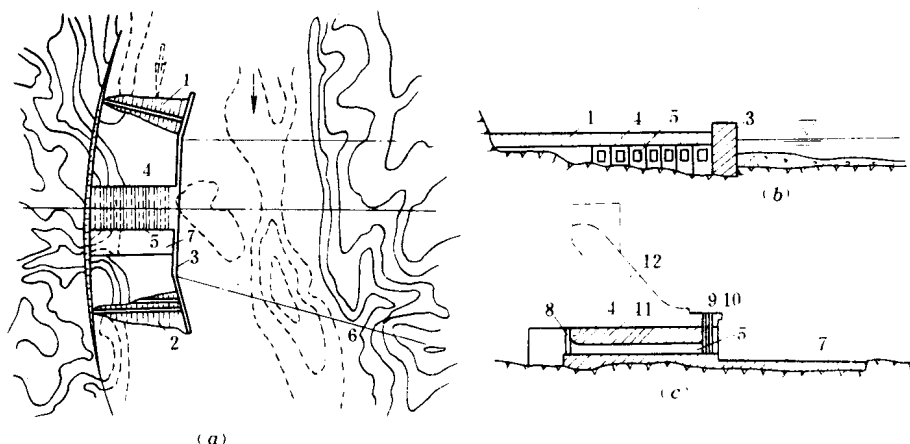
图 1-1 分段围堰法导流
