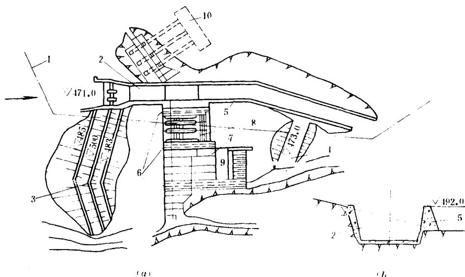
图 1-4 四川省龚嘴水电站明槽导流
