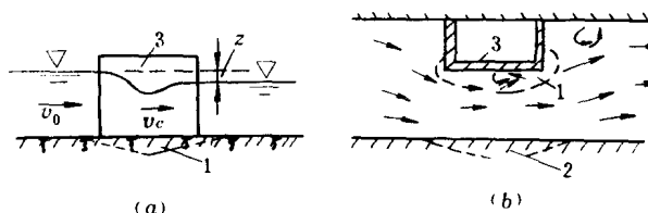
图 1-3 分段围堰束窄段水力计算图
