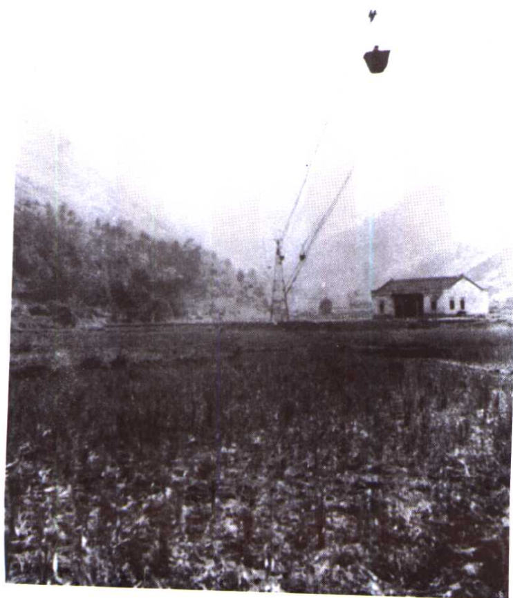
民国二十三年(1934)7月竣工的湖北大冶利 华煤矿股份有限公司空中“挂线”(运煤缆 车)(全长4500m)
