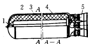
图 1-13 火药在弹道式导弹（民兵 IV）第一、二、三级发动机中的应用
