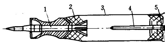
图 1-7 火药在 120mm 高压滑膛炮 脱壳穿甲弹中的应用
