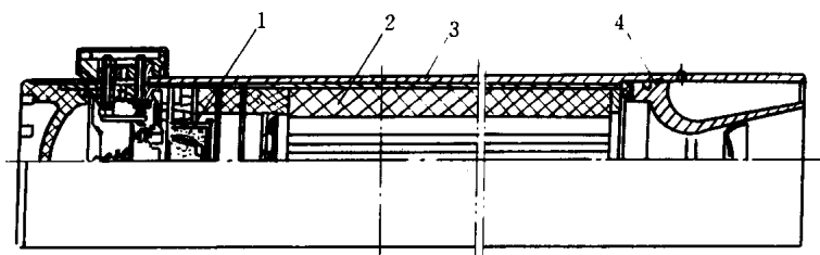
图 1-11 火药在空空导弹发动机中的应用
