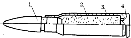
图1-1 火药在枪弹中的应用
