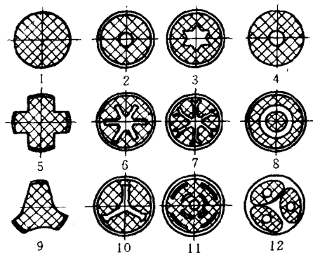
图 1-18 某些火箭火药柱的端面形状
