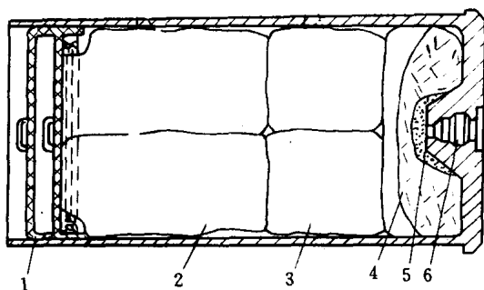
图 1-4 火药在 122mm 火炮榴弹药筒中的应用
