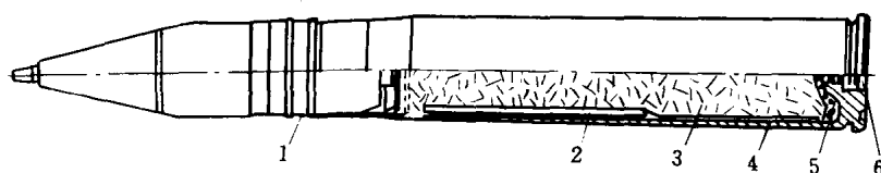
图 1-2 火药在 37mm 高炮榴弹中的应用
