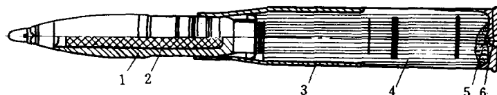
图 1-3 火药在 100mm 高炮榴弹中的应用
