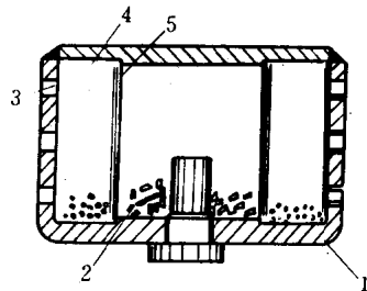
图 1-16 火药在汽车驾乘人员安全防撞装置中的应用 1—壳体；2—火药；3—排气孔；4—气体冷却与过滤室；5—过滤网
