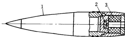
图 1-8 火药在 155mm 火炮底部 排气弹中的应用 1—弹丸；2—点火药；3—火药
