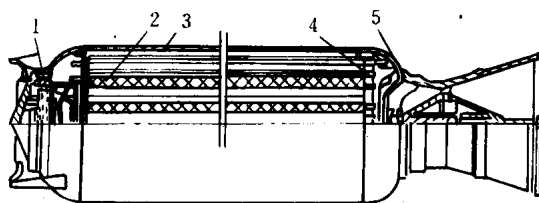
图 1-12 火药在防空导弹助推器中的应用
