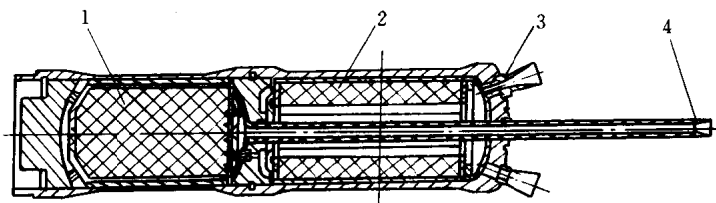
图 1-10 火药在反坦克导弹中的应用
