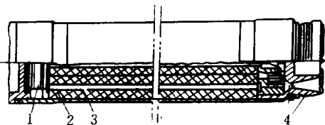
图 1-9 火药在野战火箭弹发动机中的应用 1—点火药；2—管状火药；3—燃烧室壳体；4—喷管
