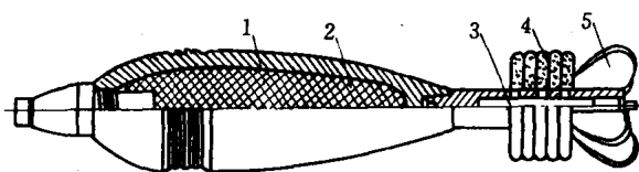
图 1-6 火药在 100mm 迫击炮弹中的应用
