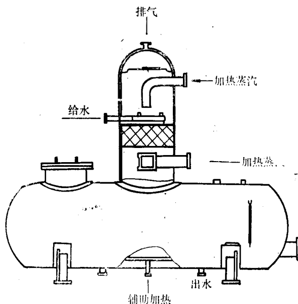
除氧器结构简图
