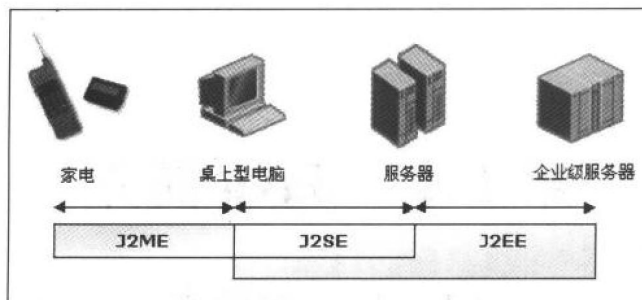
图 1.1 Java 的版本
