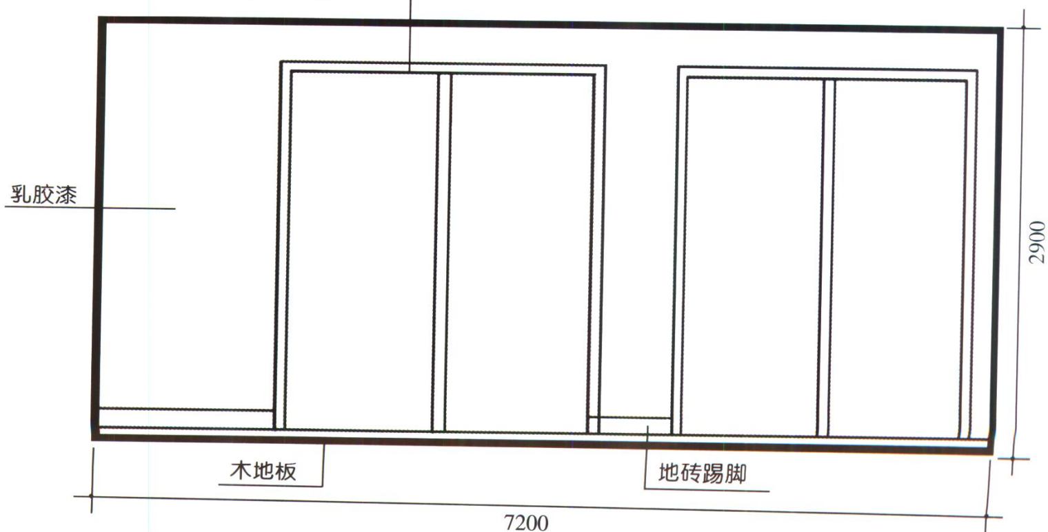
落地门窗
