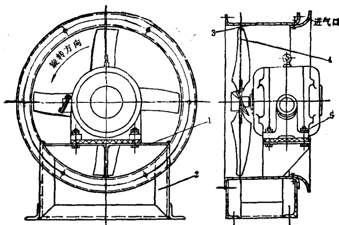
图7-1-3 低压轴流通风机
