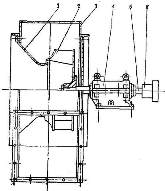
图7-1-1 中低压离心通风机
