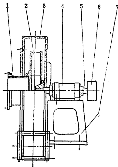
图7-1-2 高压离心通风机
