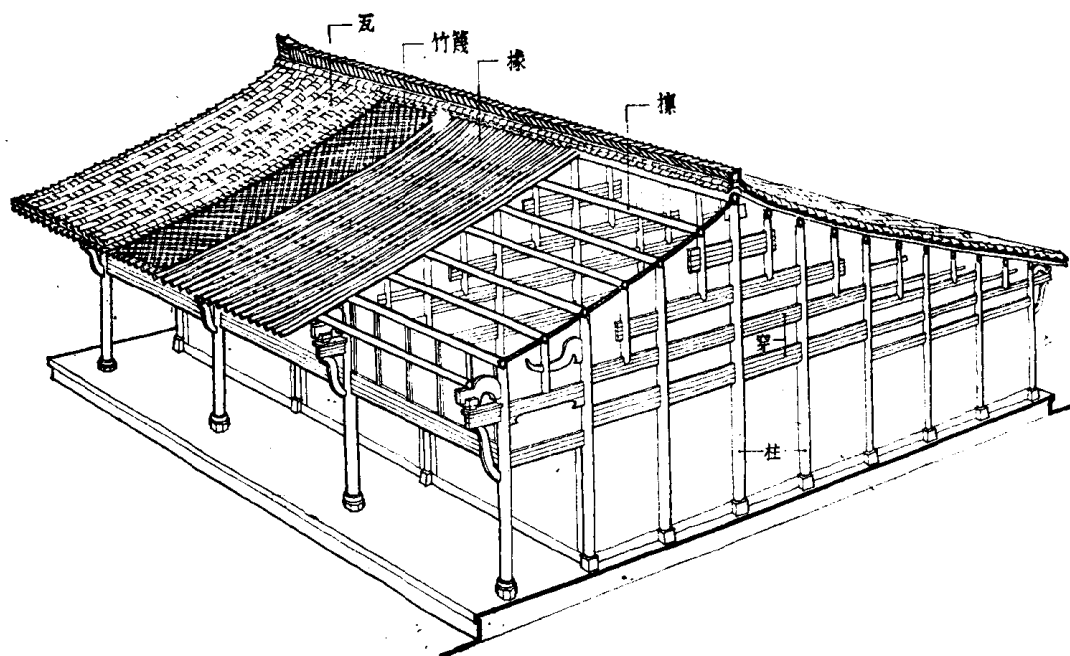
1—2 穿斗式木构架
