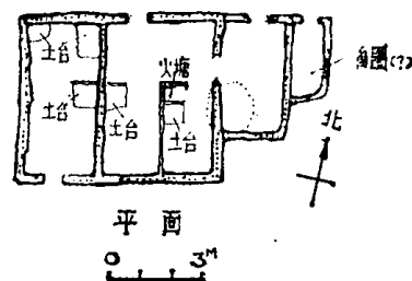
5—5 郑州大河村遗址 F 1-4
