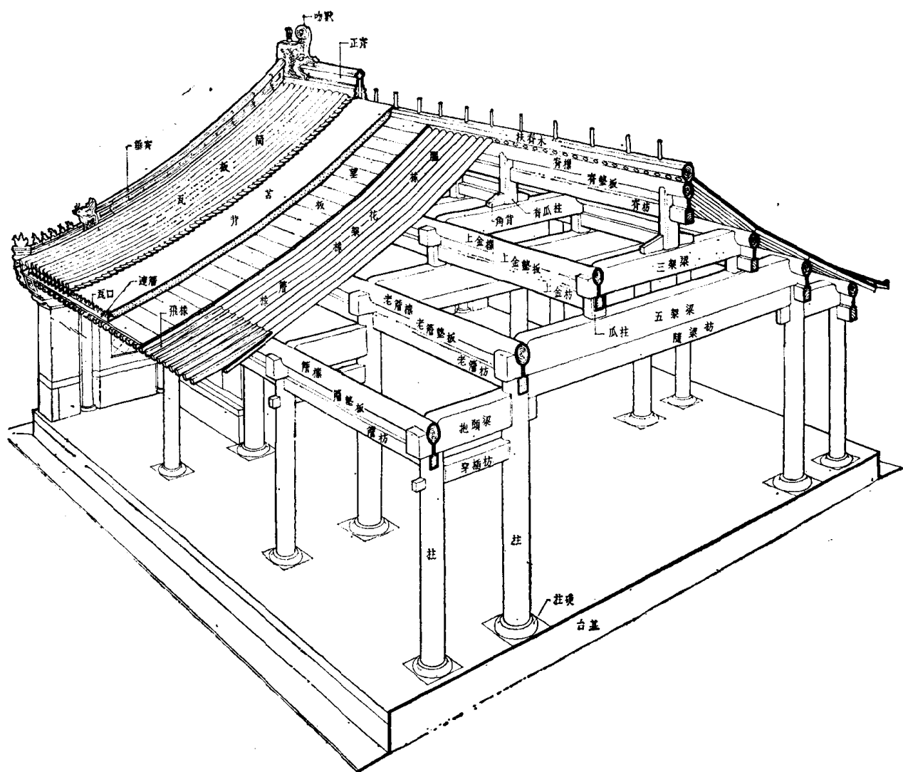
1—1 清式建筑木构架
