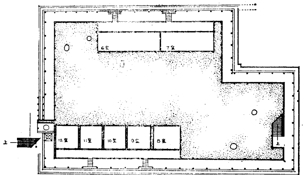
底层复原平面
