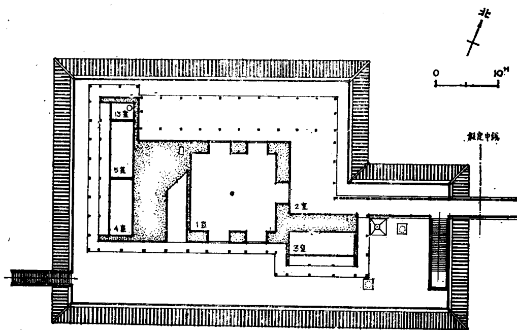
二层复原平面
