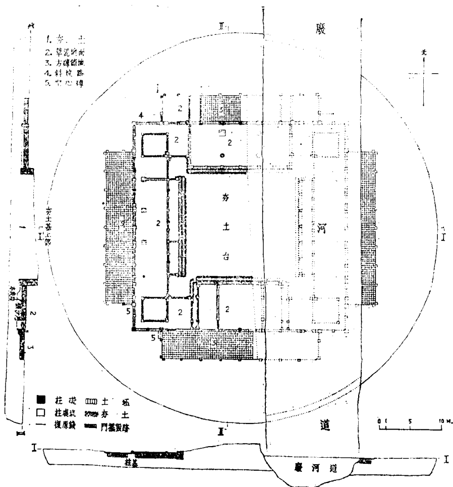
12—1 漢長安南郊禮制 建築遺址平面圖
