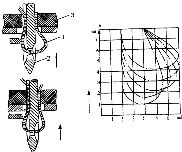
图1-2 机针的线环形成和线环的宽度变化
