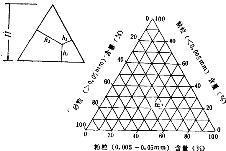
图1-3 三角坐标表示粒度成分
