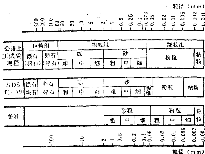
图1-1 土粒粒组的划分
