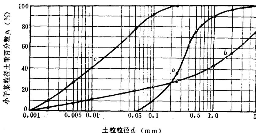
图1-2 粒度成分累计曲线
