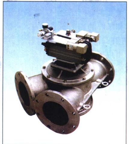
输送换向阀
