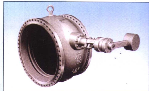
重锤缓闭止回阀
