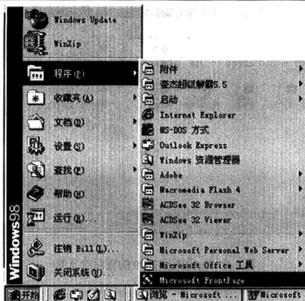
图 2-4 FrontPage 2000 运行图
