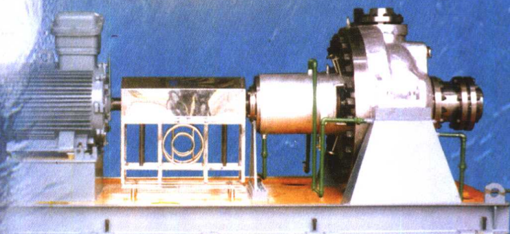
ZPY 型全衬里油浆泵: 该泵适用于炼化厂催化裂化装置。属国家专利产品。流量: 40 \sim 1000 \text{ m}^3/\text{h} , 扬程: 70 \sim 210 \text{ m} , 工作温度: < 420^\circ\text{C} 。
