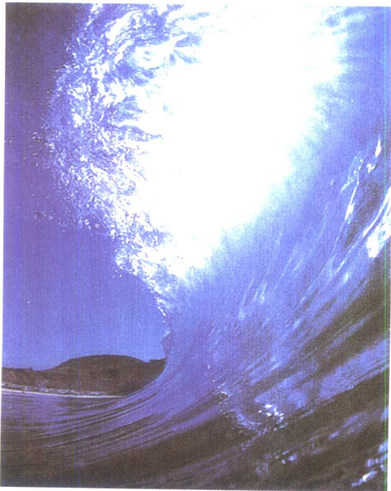
拍岸浪
