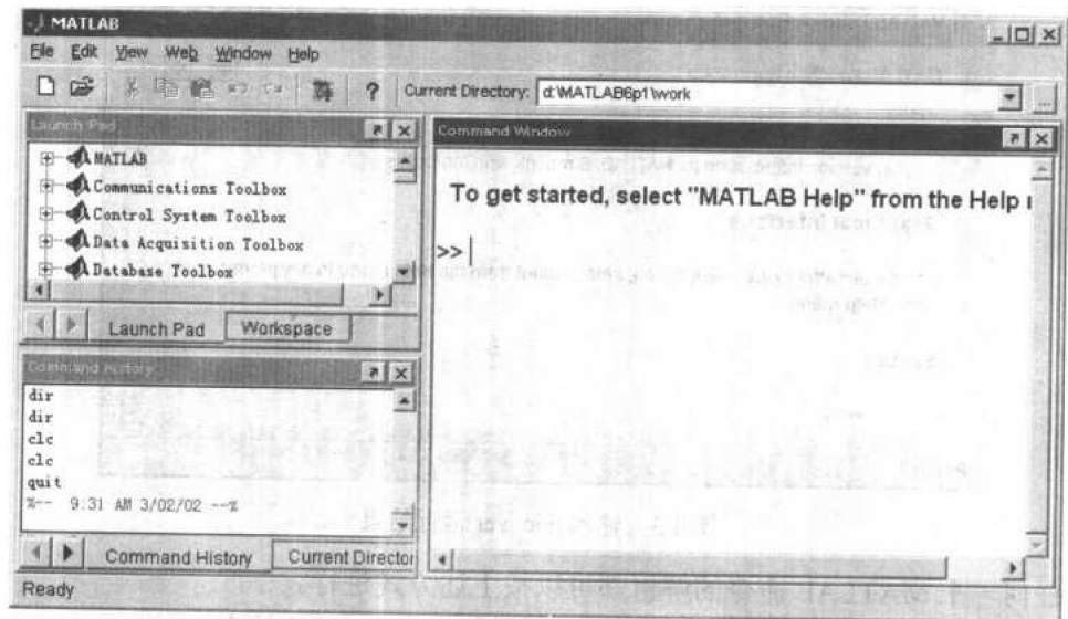
图 1.5 MATLAB 界面
