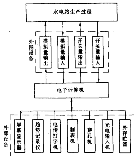
图 1-1 计算机控制系统示意图
