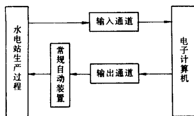
图 1-4 监督控制示意图
