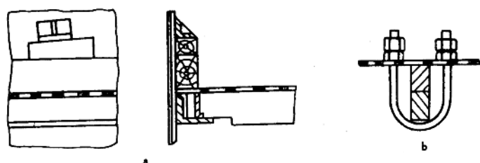
图 1-10 筛板的固定方法
