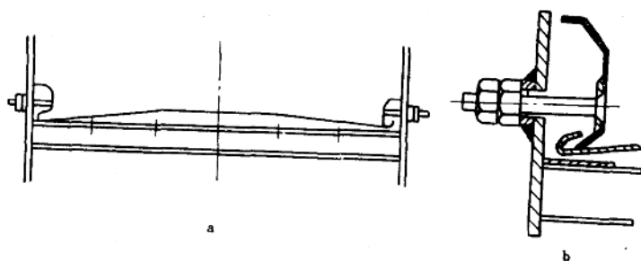
图 1-12 金属筛网的固定方法
