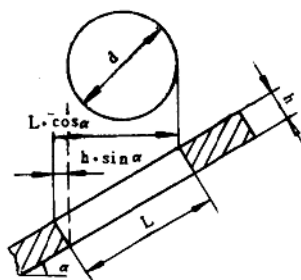
图 1-8 颗粒穿过倾斜筛面的筛孔示意图
