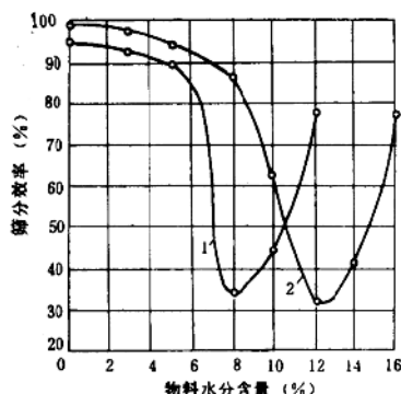
图 1-6 筛分效率与物料湿度的关系 1—吸湿性弱的物料；2—吸湿性强的物料
