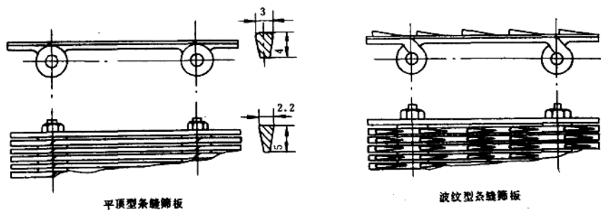
图 1-14 条缝筛面的筛条形状
