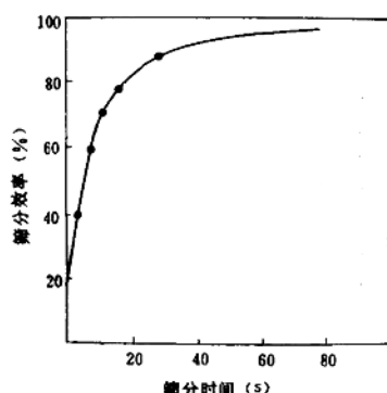
图 1-7 筛分效率与筛分时间的关系
