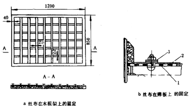
图 1-13 网状丝布的固定方式
