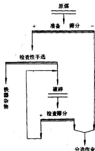
图 1-2 原煤准备工艺流程
