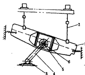
图 1-1 WK型振动筛
