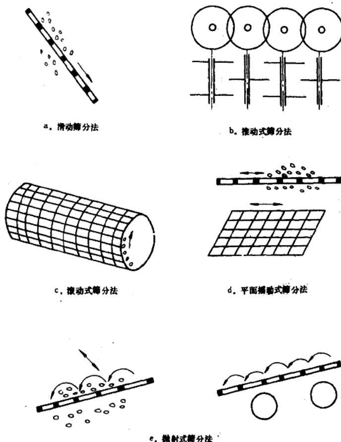
图 1-3 各种筛分方法
