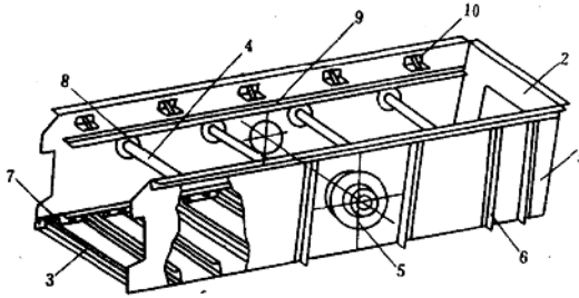
图 1-9 筛框的结构
