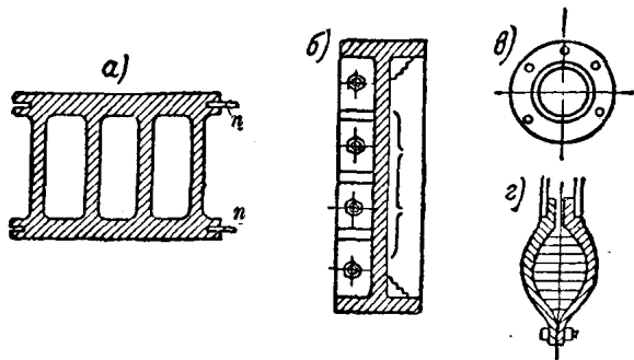
圖 2 生鐵拱塊截面式樣
