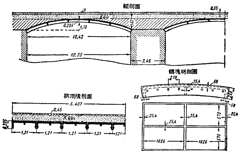
圖 3 膈梗式生鐵塊拱橋構造（土拉城烏河橋）
