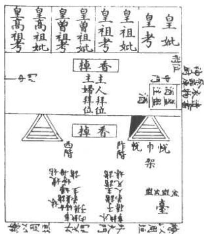
家廟、祠堂圖
