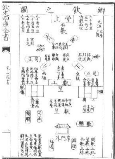
乡饮图
