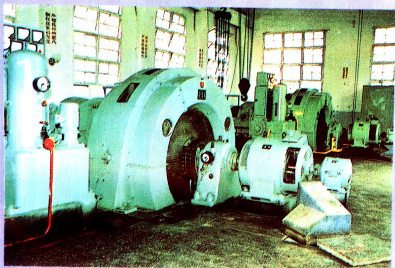
▼涪陵地区土坎发电厂二级站水机室
