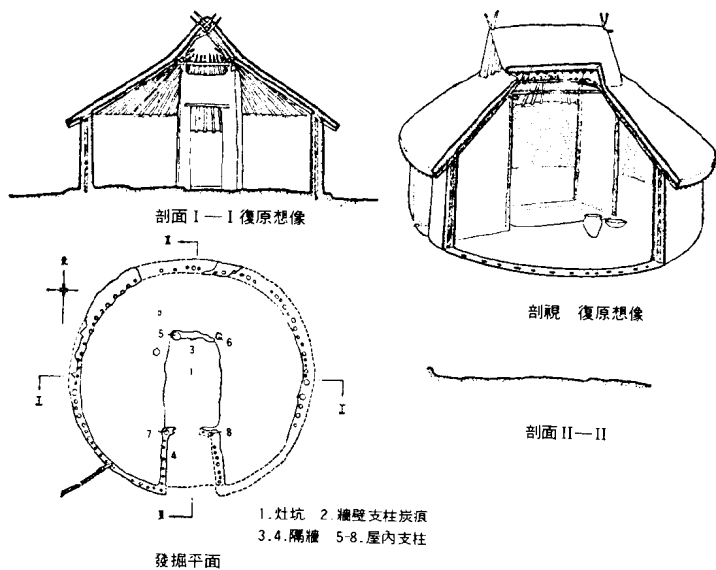
圖 2 圓形住屋
