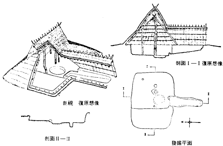
圖 1 方形住屋
