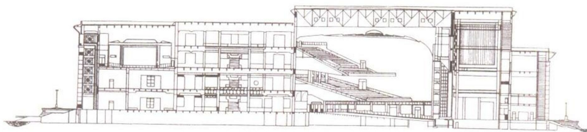
2. 剖面图
