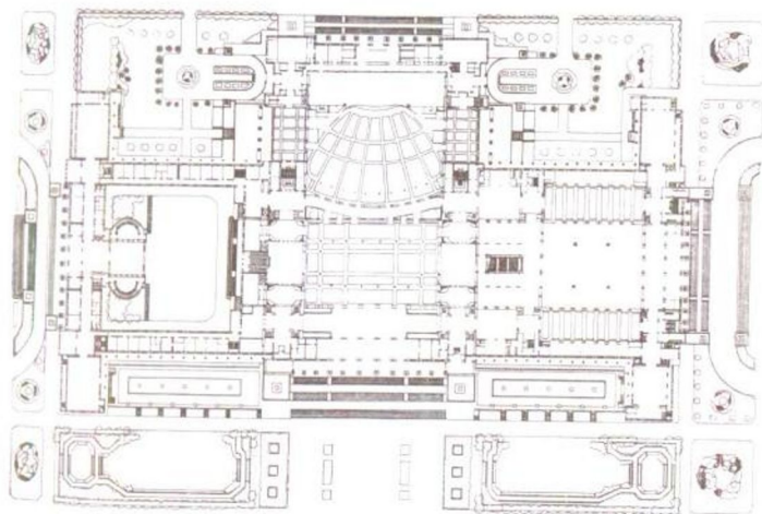
3. 首层平面图
