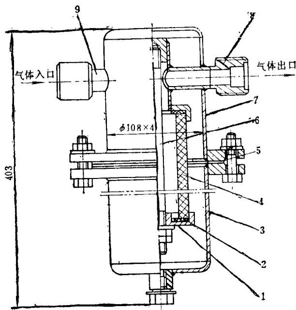
图11-7 陶瓷管过滤器
