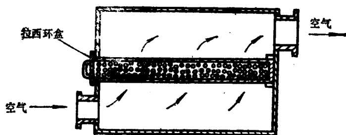
图11-3 拉西环过滤器
