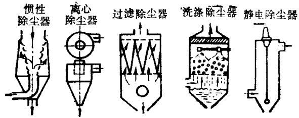
图11-1 几种除尘装置示例
