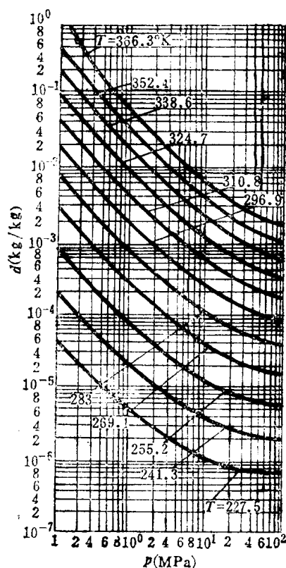
图11-9 不同压力下压缩空气 中饱和含湿量
