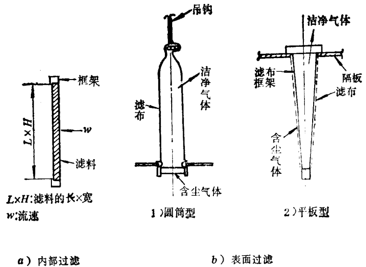
图11-2 过滤除尘的过滤方式
