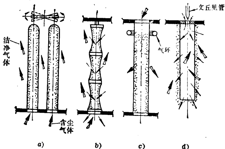
图11-6 清灰机构
