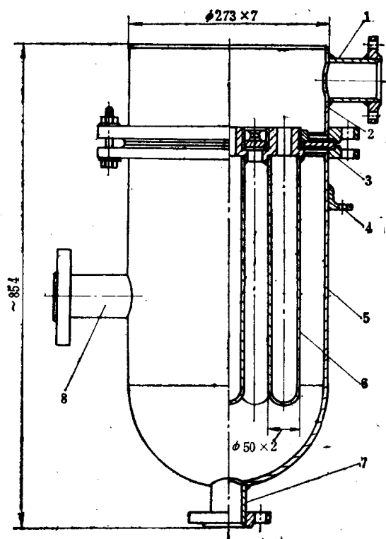
图11-8 粉末冶金管过滤器
