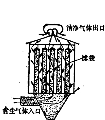
图11-5 袋式过滤器
