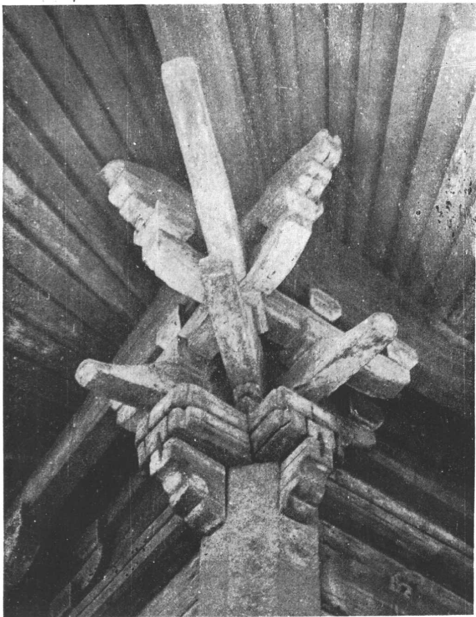
甲 三清殿下簷轉角鋪作(其一)
