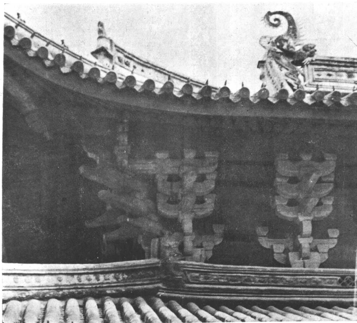
作鋪角轉簷外簷上殿清三 丙
