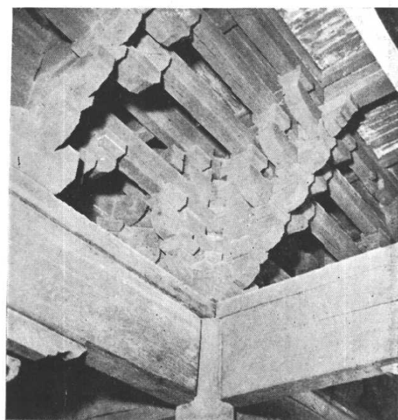
甲 三 清 殿 內 簷 東 第 三 斗 拱
