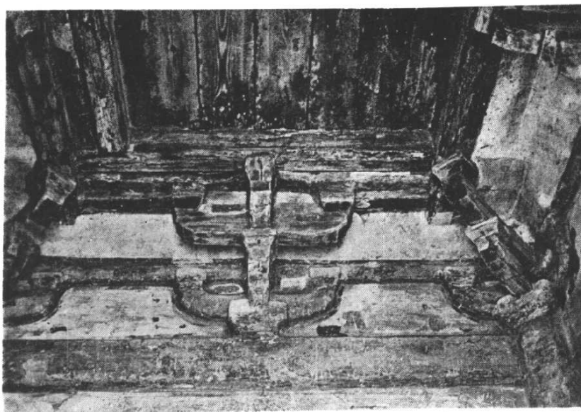
乙 西塔第一層內簷斗拱
