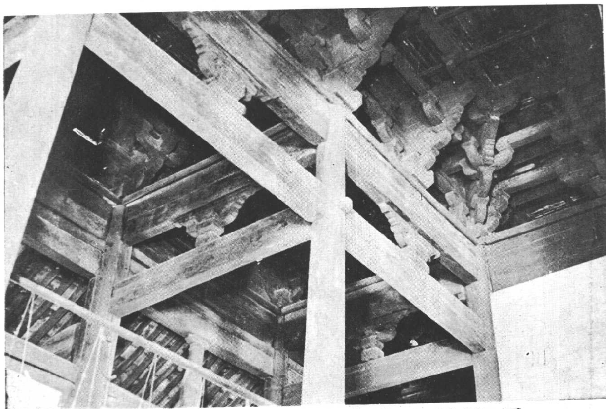
丙 三 清 殿 內 簷 西 第 三 縫 及 梢 間 梁 架
