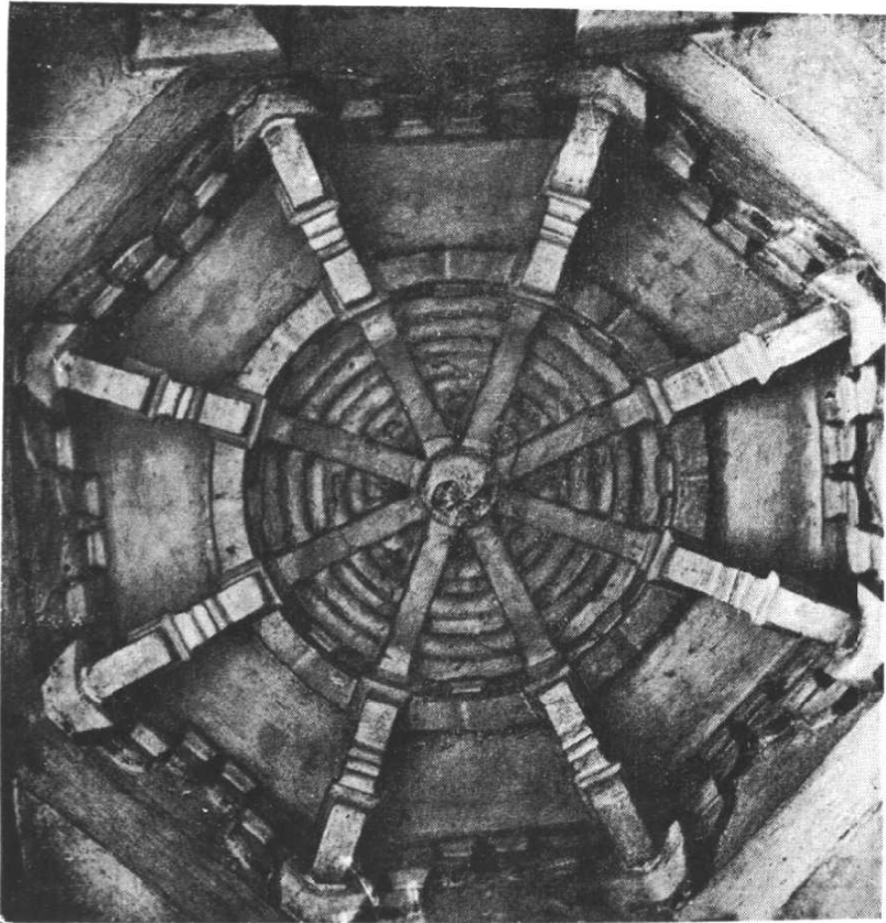
甲 報恩寺塔塔心走道
