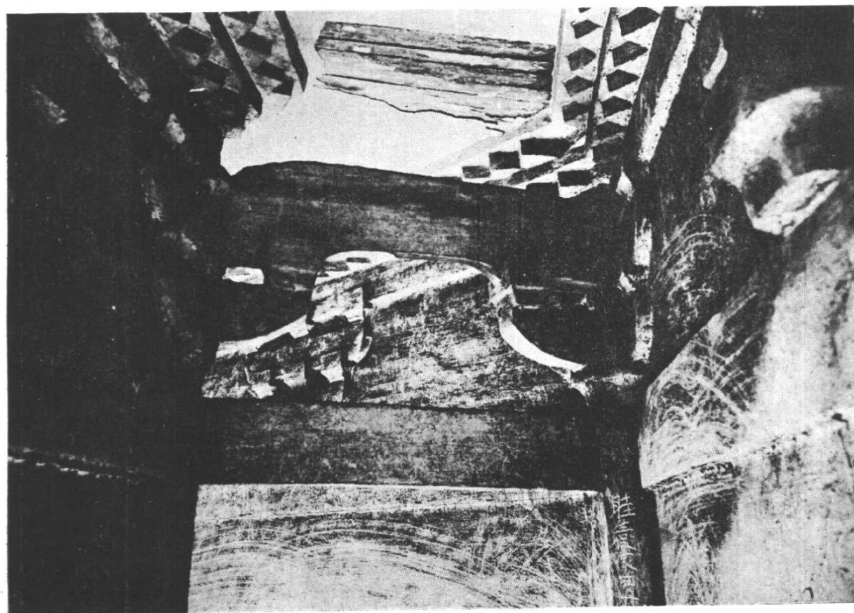
構結廊內層二第塔寺恩報 乙
