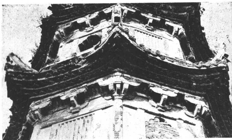
甲 西塔第二層外簷斗拱
