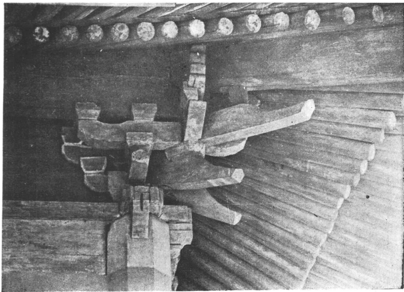
乙 三清殿下簷轉角鋪作(其二)
