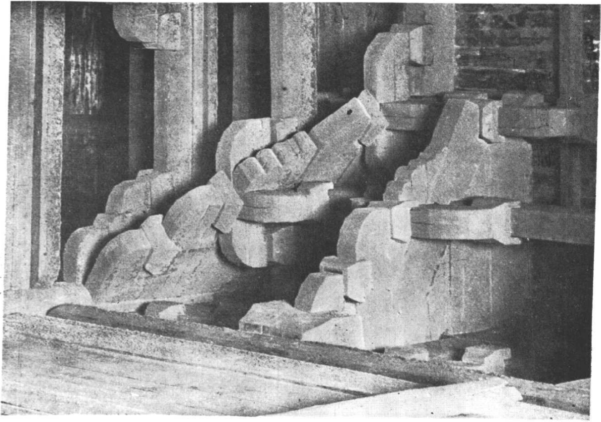
乙 三清殿內簷當心間斗拱詳部
