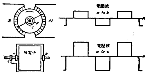
第一圖 電壓波之一
