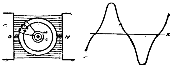
第二圖 電壓波之二
