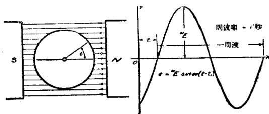
第三圖 電壓波之三
