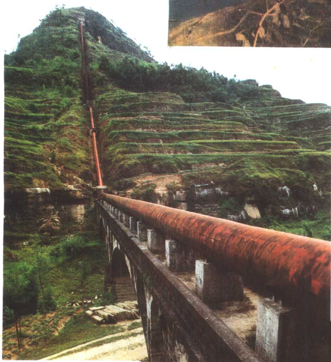
友谊水库干渠倒虹管
