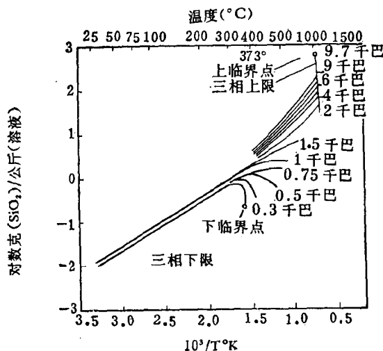
图 1-3 水中石英的溶解度综合图解(据贺伦)
