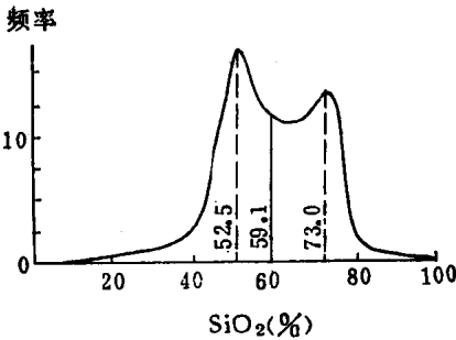
图 1-1 火成岩中硅氧分布的频率 (据仿巴什, 1962)
