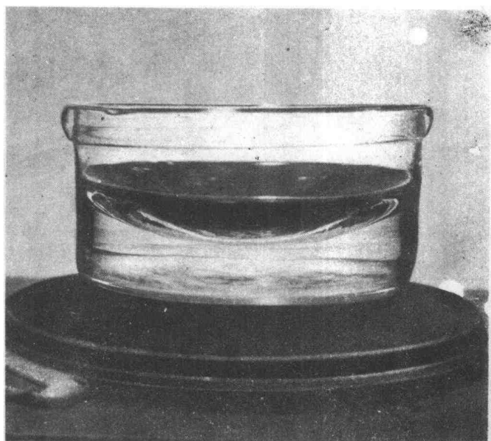
轉動的水所成的拋物面
