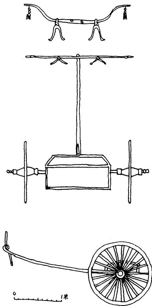
陕西长安西周早期车的复原图
