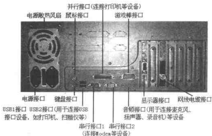
图1-4 机箱背部面板
