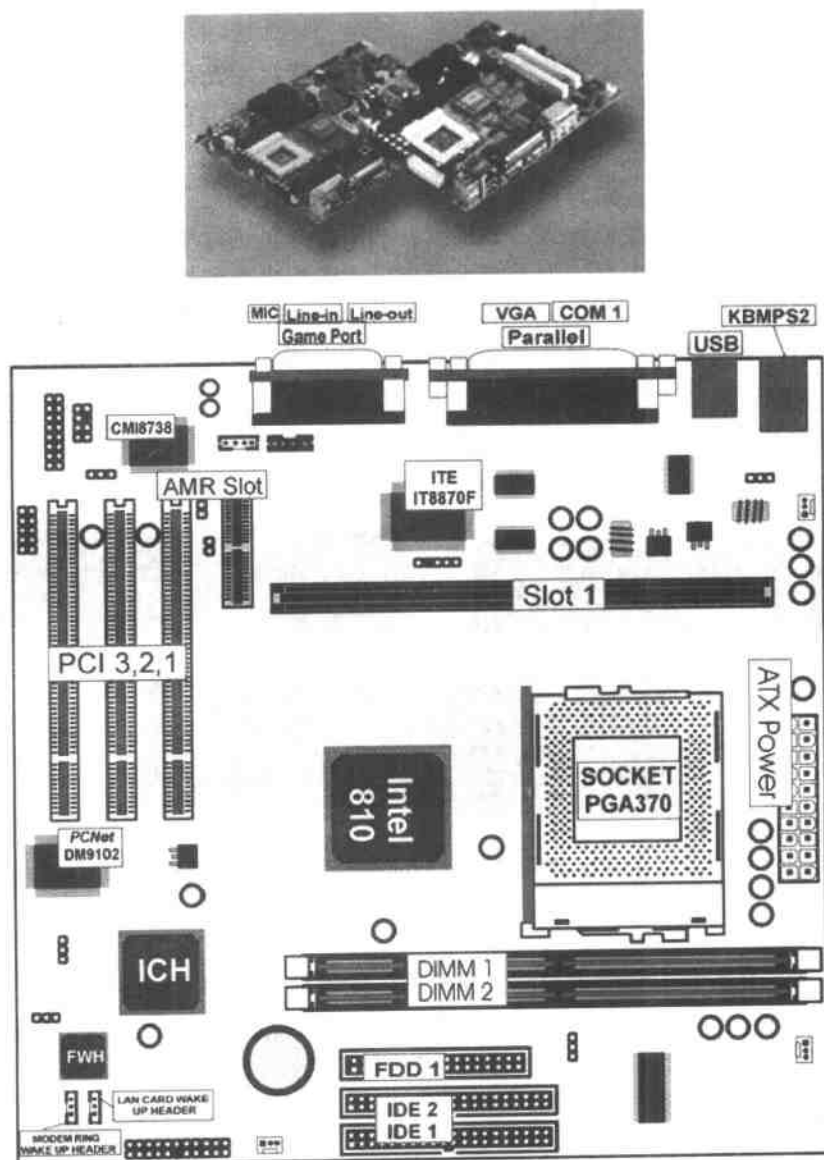
图1-5 主板
