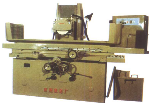
杭州机床厂生产的“部优”产品 MG7132A 精密卧轴矩台平面磨床
