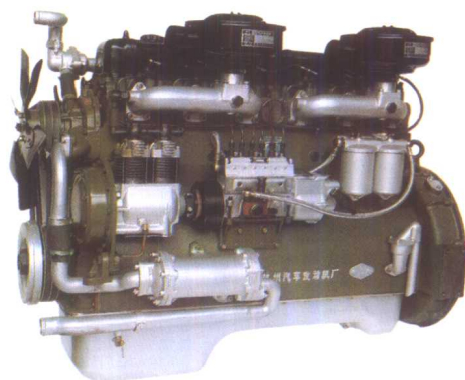
杭州汽车发动机厂生产的 6120 型 柴油机获“部优”产品称号
