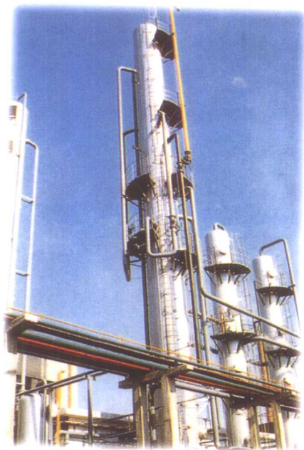
杭州市化工研究所 1978 年研制成功 碳酸丙烯酯脱除二氧化碳新工艺
