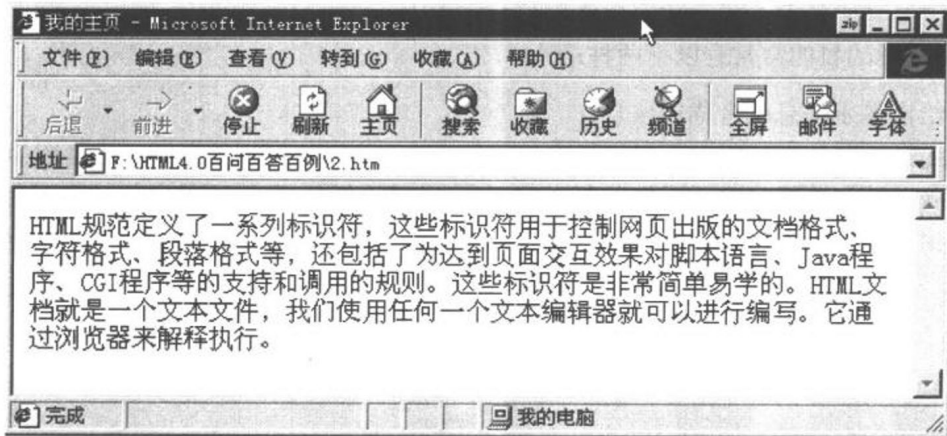
图 1.3 HTML 文档
