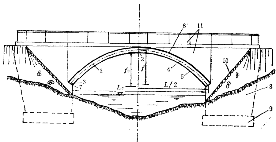
图4-1-4 实腹拱桥
