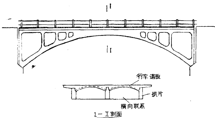
图4-1-8 拱片桥
