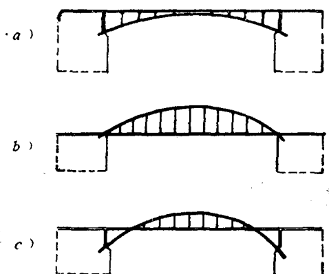
图4-1-3 上承式、下承式及中承式拱桥图式
