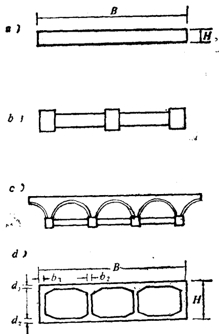
图4-1-9 拱的横截面型式 a)板拱-整块矩形实体截面; b)肋拱-分离式肋形截面; c)双曲拱-截面由数个小拱组成; d)箱形拱-整块空心箱截面
