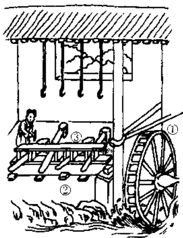
图 1-4 舂米
