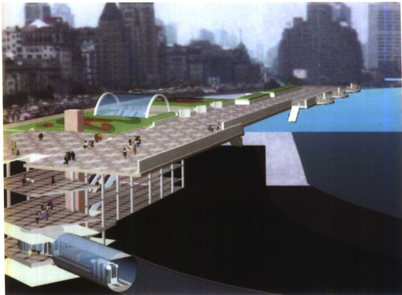
外滩观光隧道剖面示意
