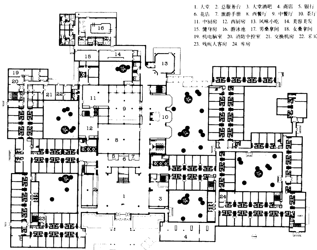
首层平面图
