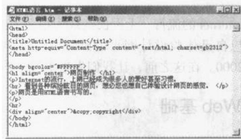
图 1-4 上面网页的 HTML 源文件
