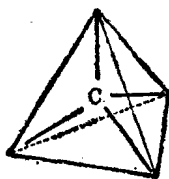
正四面体 [2]
