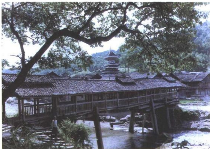
照片10 侗寨风雨桥 (贵州省丛江县信地乡往洞寨, 吴仕忠摄)
