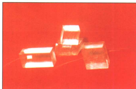
冰洲石
