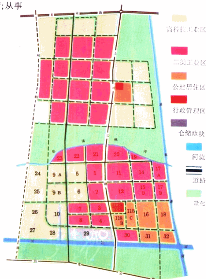
上海王桥出口工业开发区规划平面图
